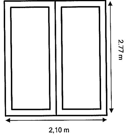
Fereastră 2 canaturi - 2 buc
